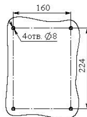
Рис.2. Установочные размеры
